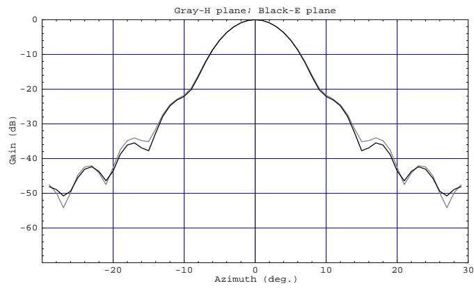
(b) 660 GHz
